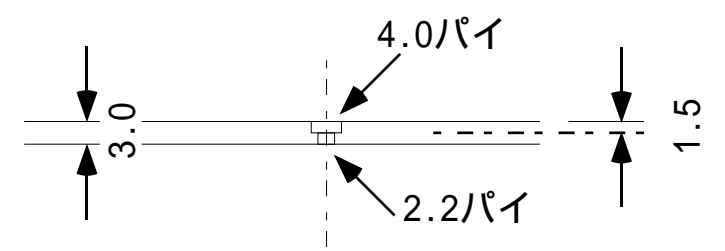
"A"孔部詳細
